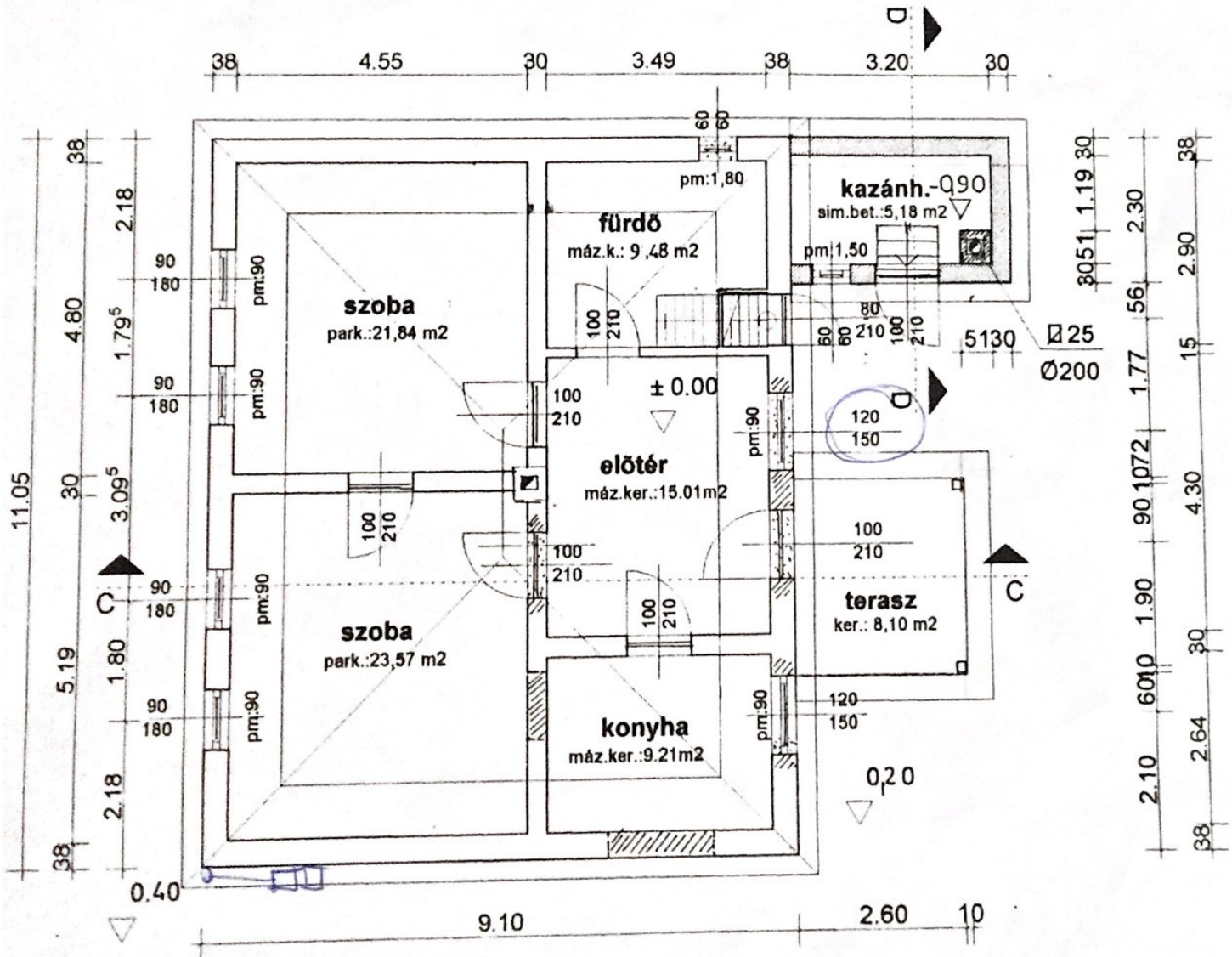
Átalakított és bővített földszinti alaprajz m 1 : 100
